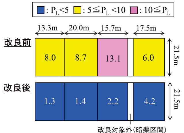
対象域の平面図とP L 値
