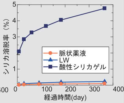
シリカ溶脱率試験結果
