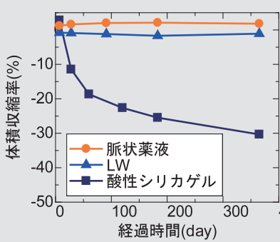
体積収縮率試験結果
