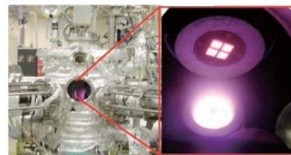
クリーンルーム内の真空チャンバー(左)と 薄膜積層中の超電導量子干渉計素子(右)
