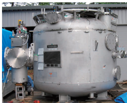
超電導磁気エネルギー貯蔵装置
