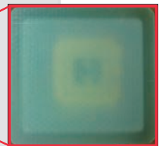
クリーンルーム内の真空チャンバー(左)と 薄膜積層中の超電導量子干渉計素子(右)
