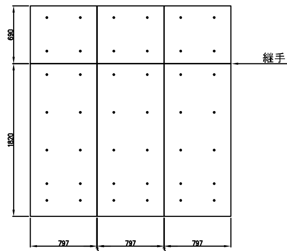
A-A側面図
