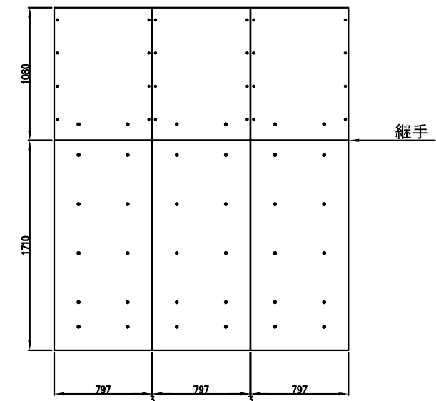
A-A側面図
