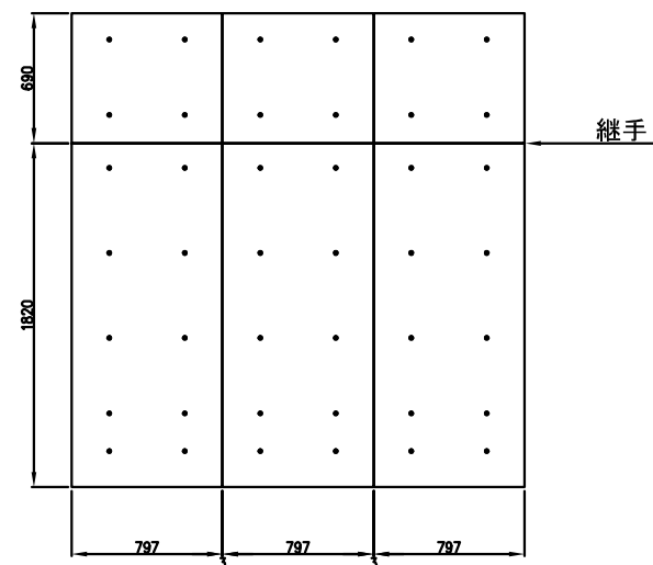
A-A側面図
