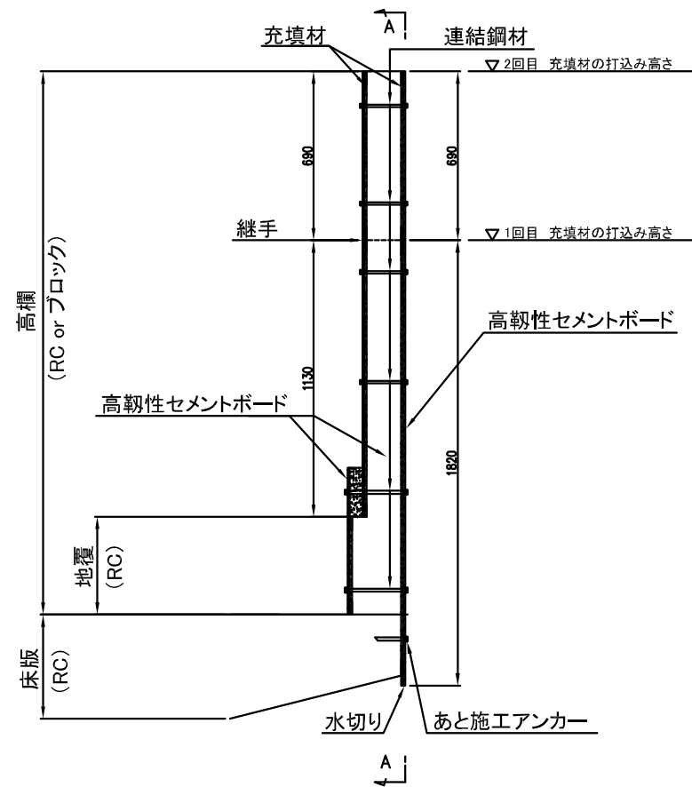
A-A側面図
