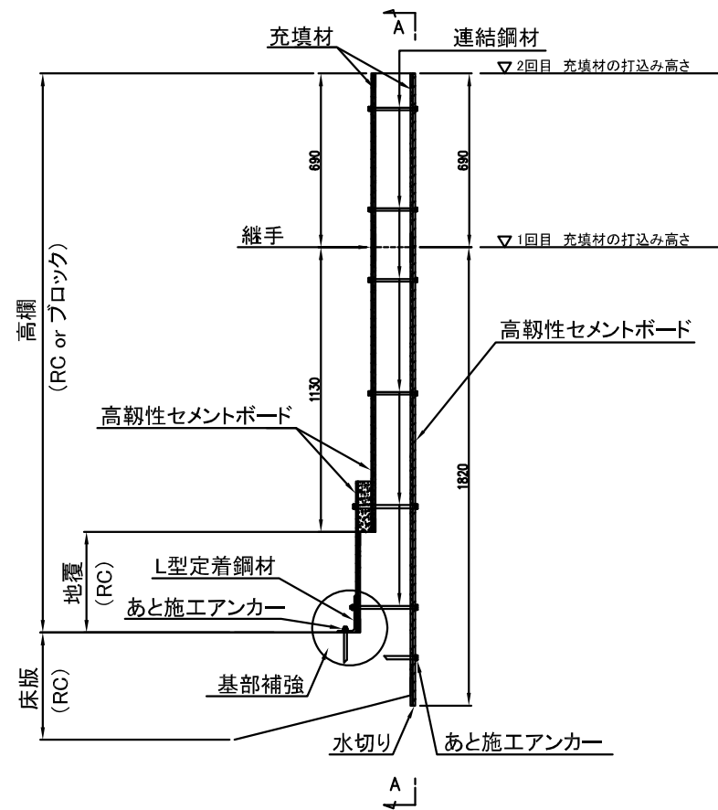
A-A側面図
