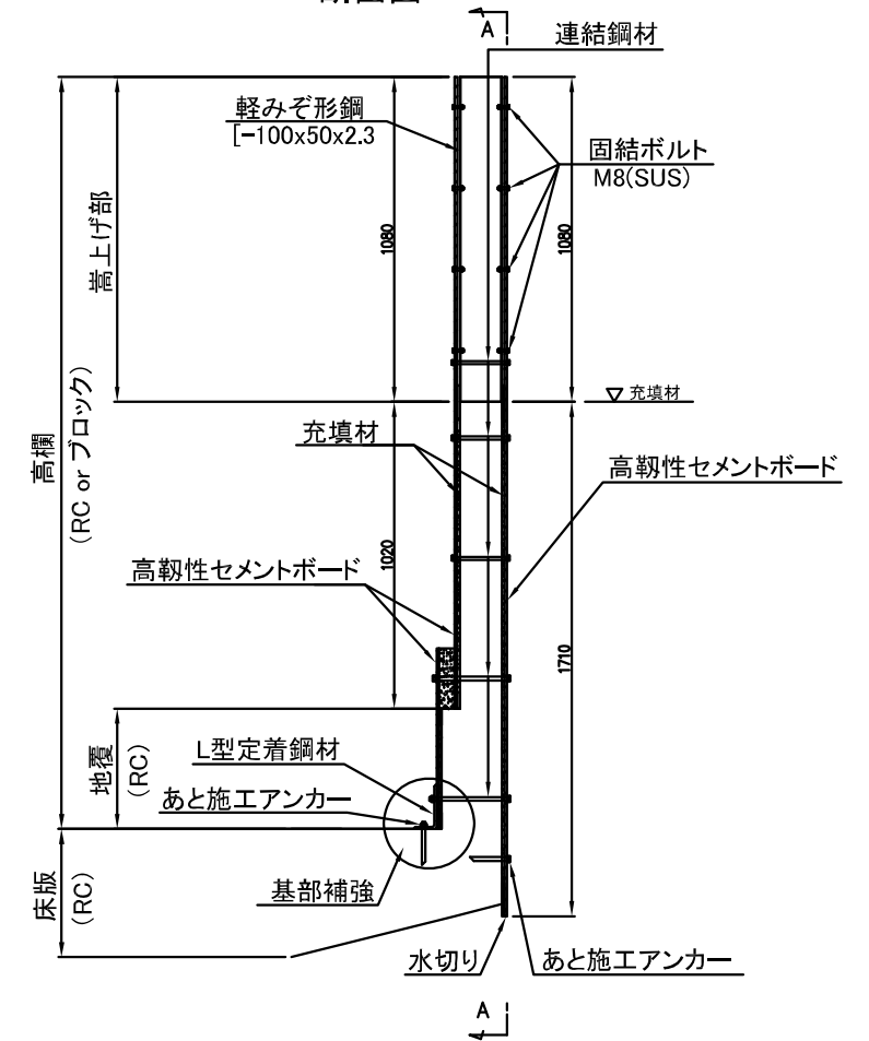
A-A側面図
