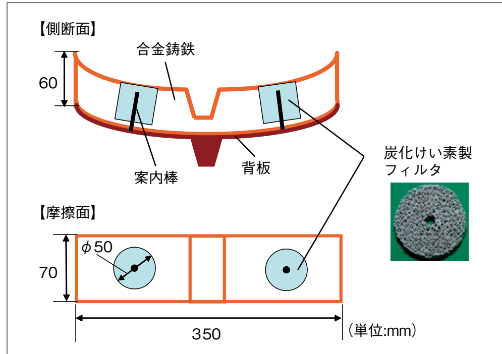
図 鋳鉄複合化制輪子の構造
