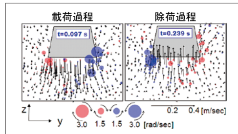
図2 まくらぎ周辺のバラスト粒子の挙動
