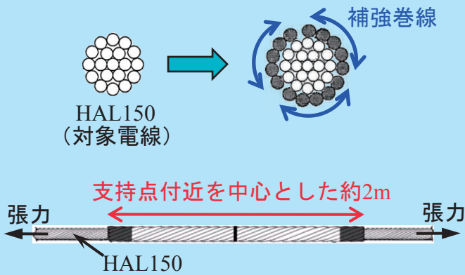
図2 補強巻線による電線・AT保護線の曲げ応力緩和機構 (HAL150の例)
