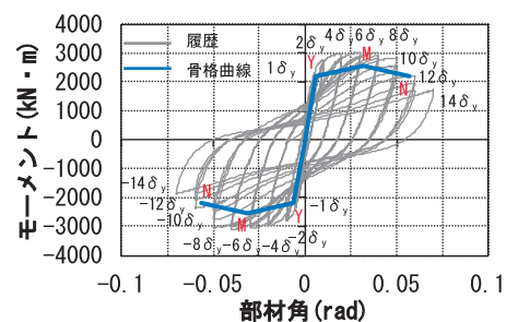
モーメント-部材角関係
