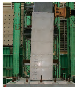
曲げ破壊実験
