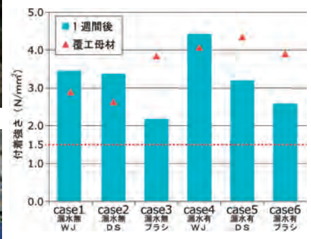
施工完了1週間後の付着強さ
