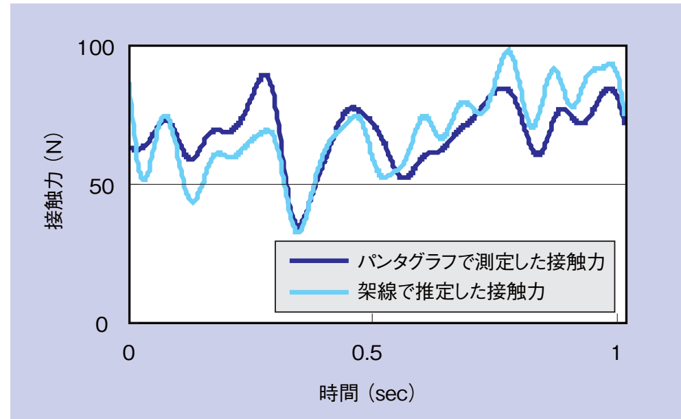
図 接触力推定結果(実験値)
