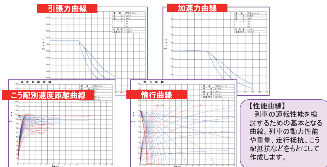
図3 性能曲線図群
