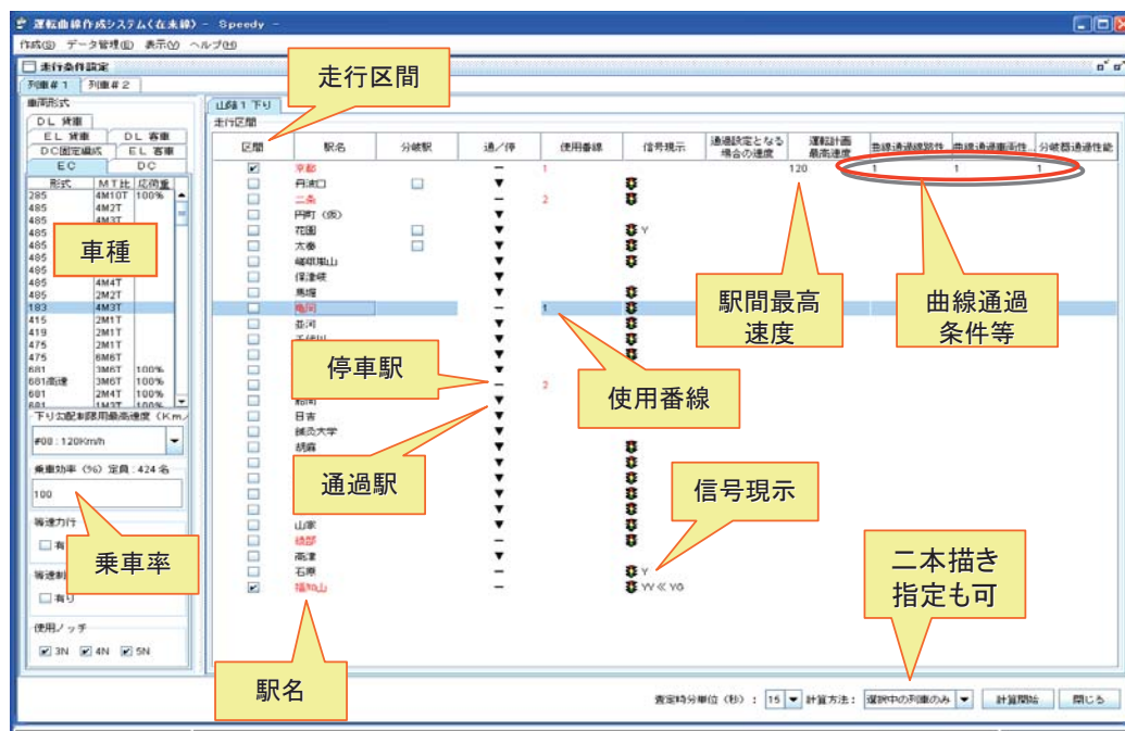
図2 走行条件指定パネルと設定項目
