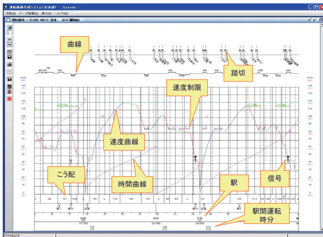
図1 運転曲線画面表示例とその内容
