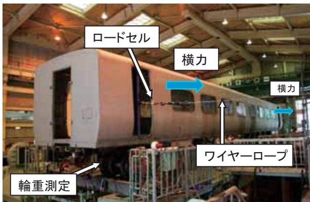
図2 動的解析式の検証試験
