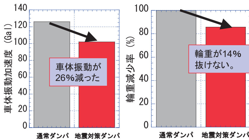
中越地震推定地震動の振幅146mm加振時の実験結果比較
