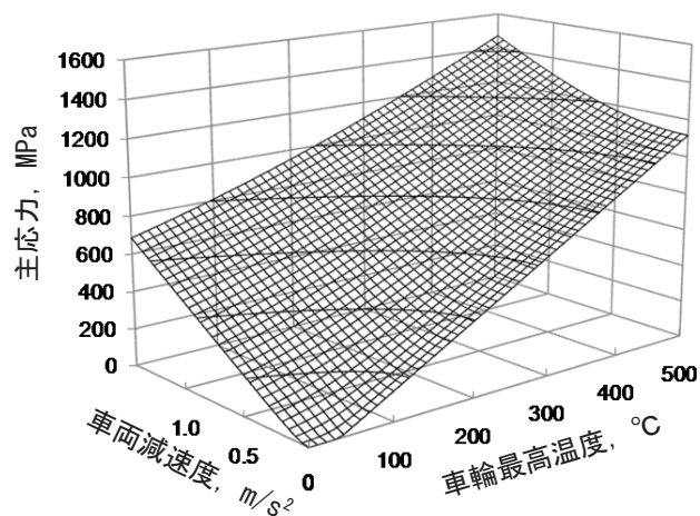
図3 熱き裂発生条件の算定法
