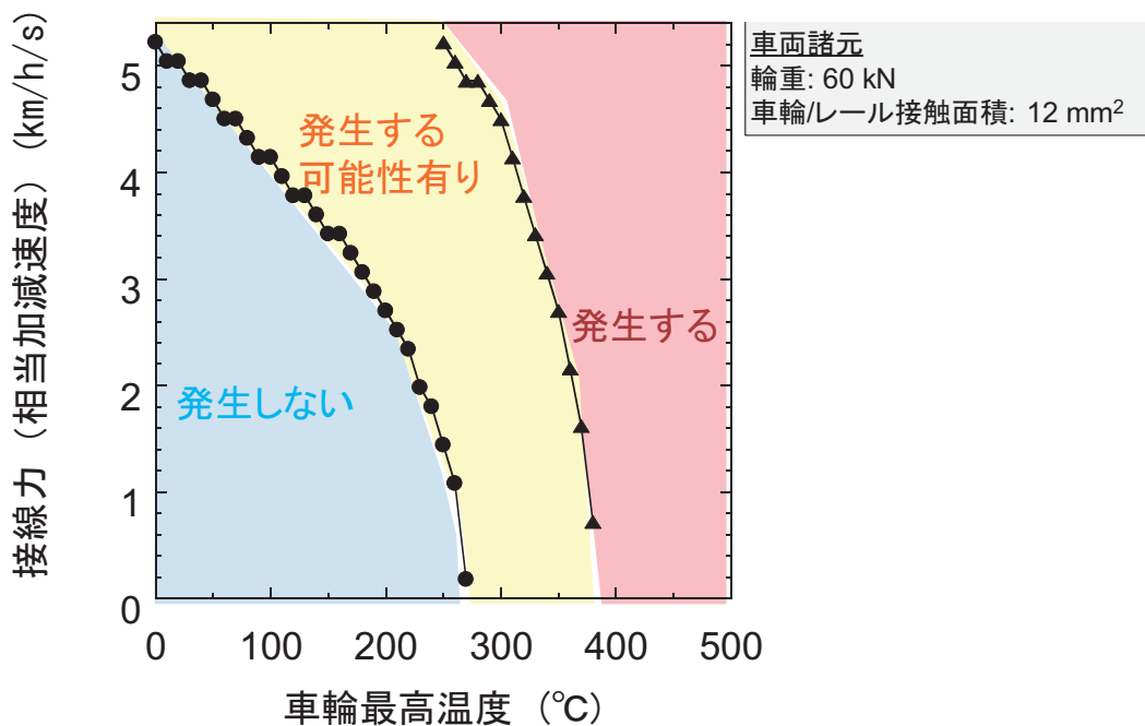
図4 踏面熱き裂発生条件指標図の例
