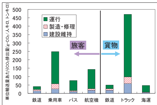
図2 産業連関表及びエネルギー統計資料による単位輸送量あたりのCO 2 排出量の比較
