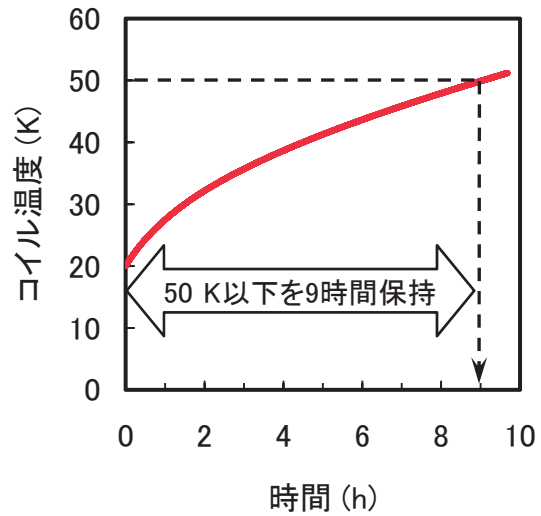
図3 保冷能力
