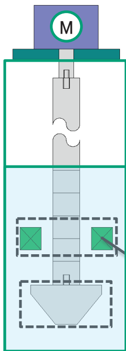
超電導ケーブル用ポンプの軸受部の構造
