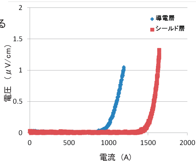
2m級Y系超電導ケーブルの通電試験結果
