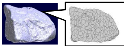
球剛接バラスト要素
