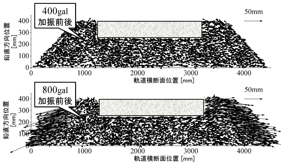
粒子移動の観察例 (解析条件: 水平加振)
