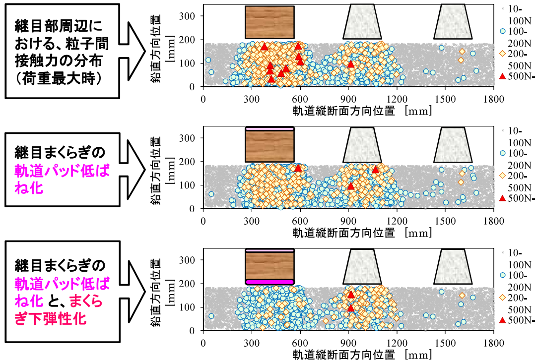
粒子間接触力の比較例 (解析条件: 継目落ち2.5mm、段差0.5mm)
