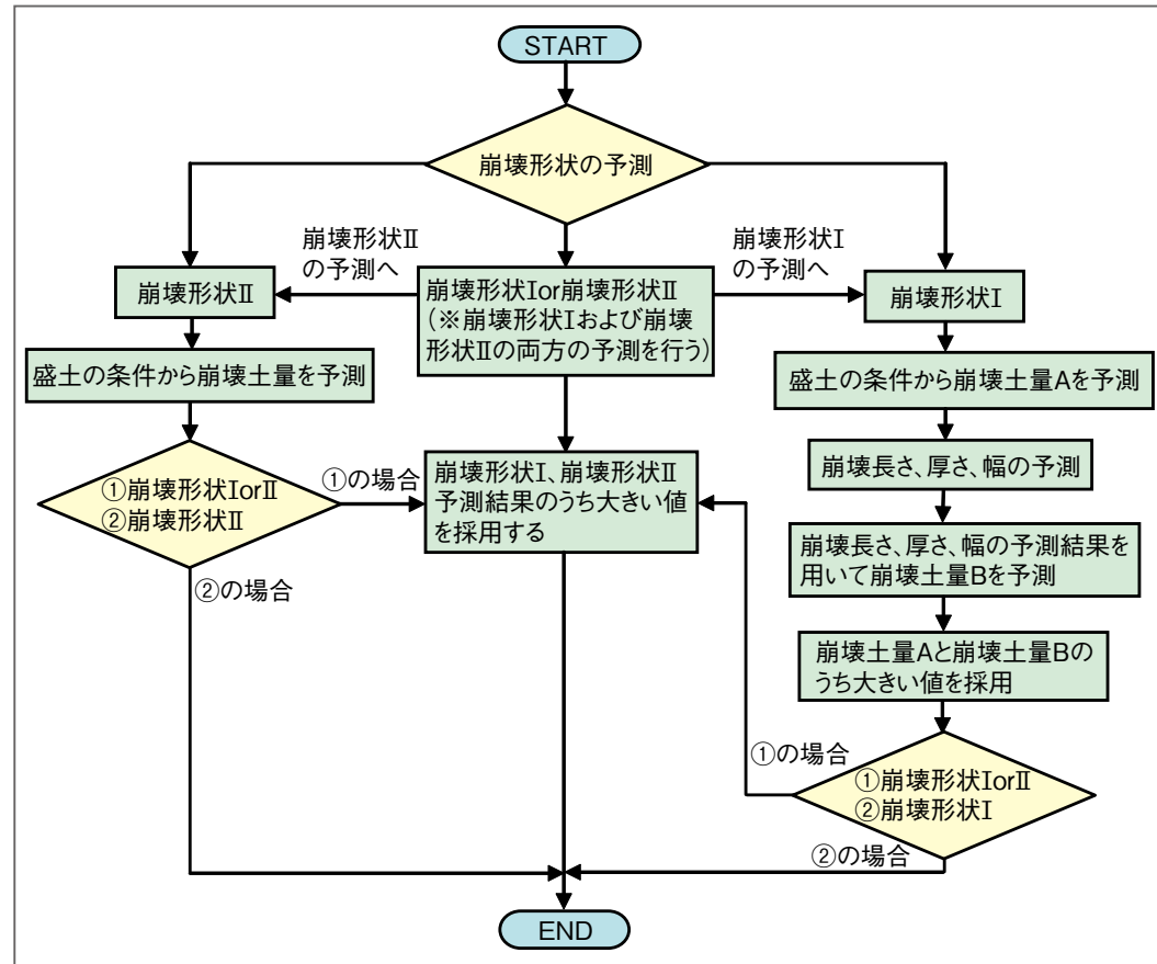
図 盛土における崩壊形状と規模の予測フロー
