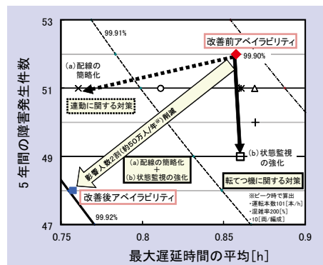
図 複数装置間での適用対策の検討 (連動装置と転てつ機に関する対策の組み合わせ)
