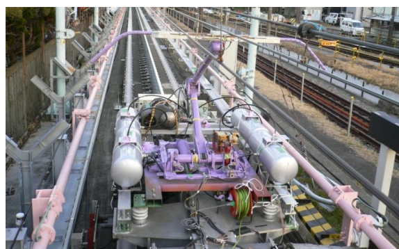
(c) アクティブ制御パンタグラフ
