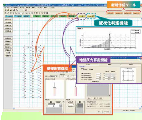
静的非線形解析の表示画面例
