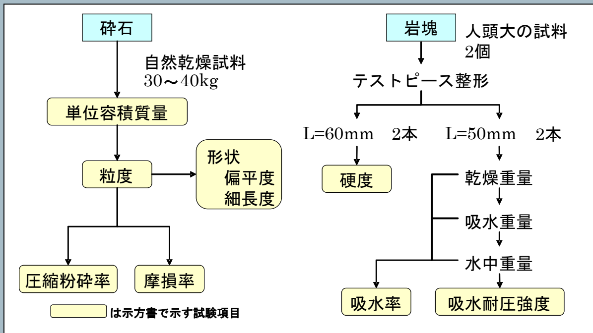
図1 道床バラスト石質試験フロー
