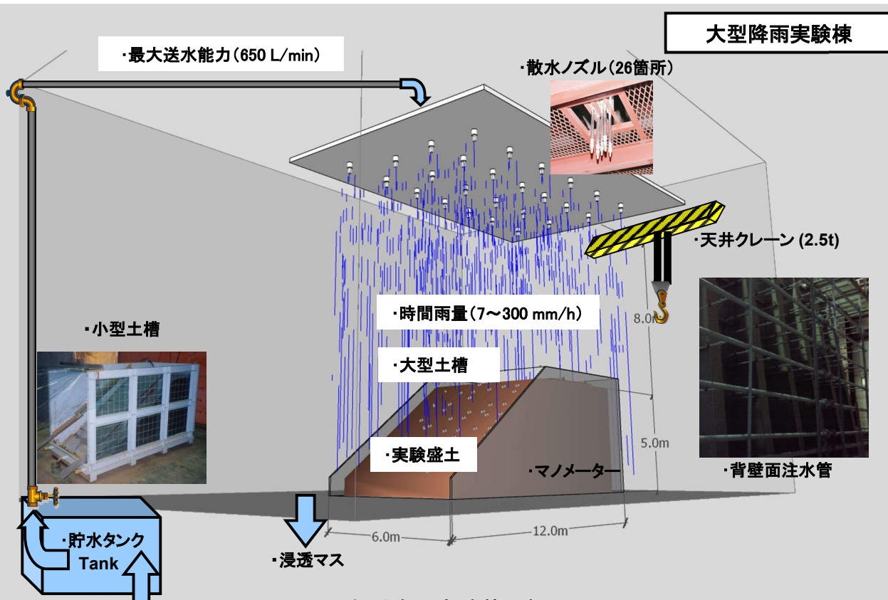
図1 大型降雨実験装置概要
